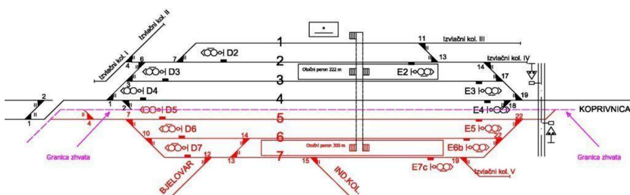
Slika 7 – Novo stanje kolodvora Križevci
