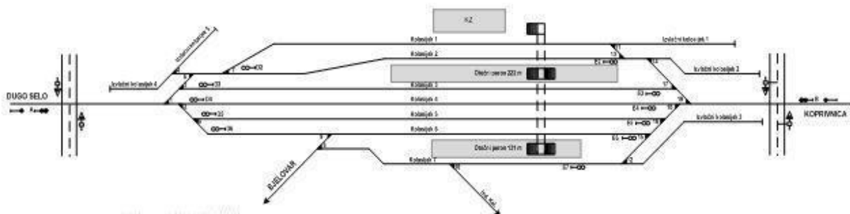
Slika 4 – Postojeće stanje kolodvora Križevci
